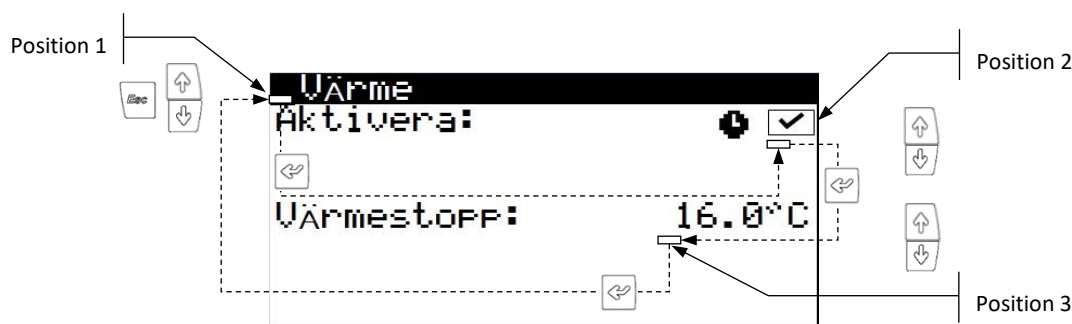
Bild 3.4. Justera komfortparametrar.
