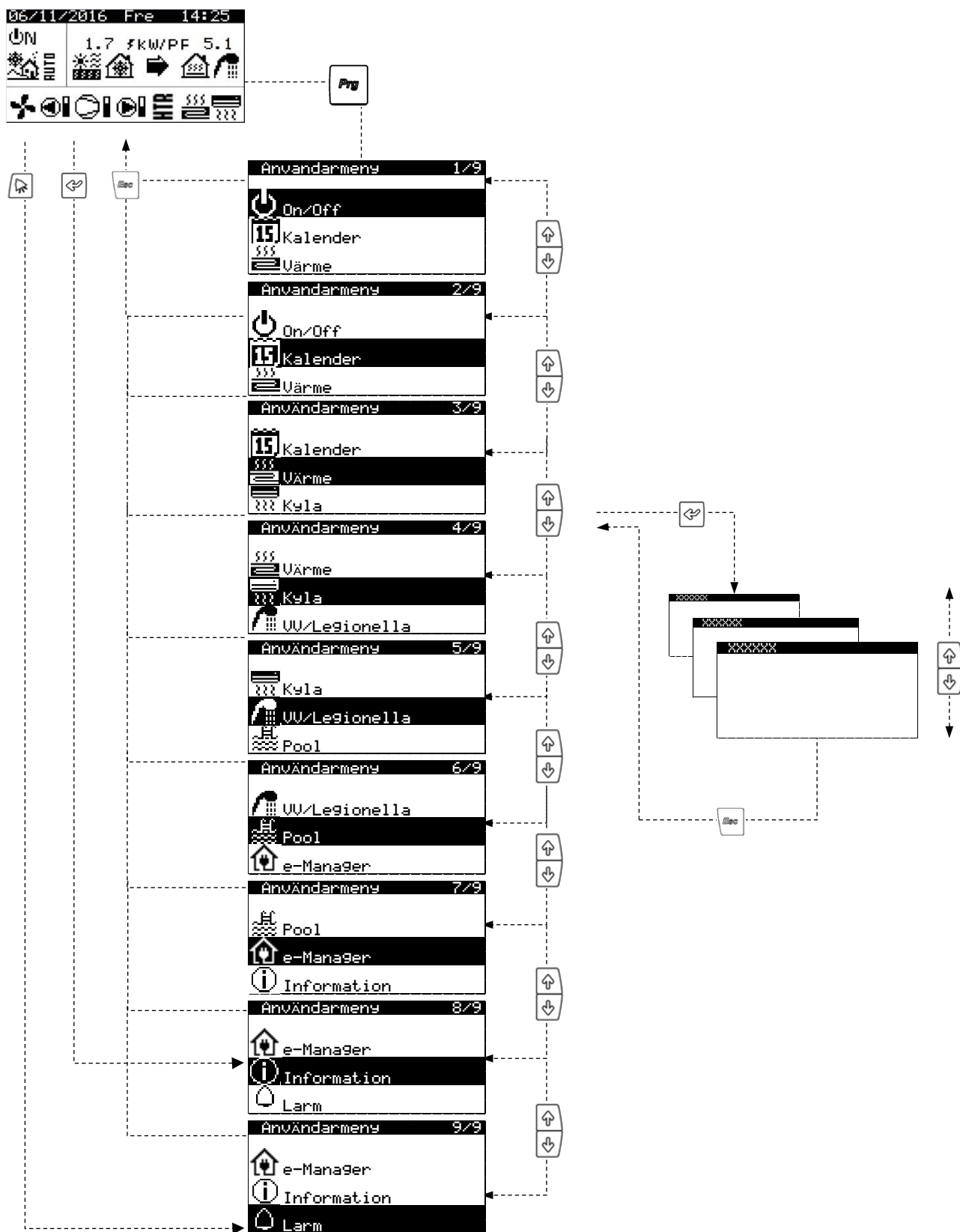
Bild 3.3. Användarmeny.
