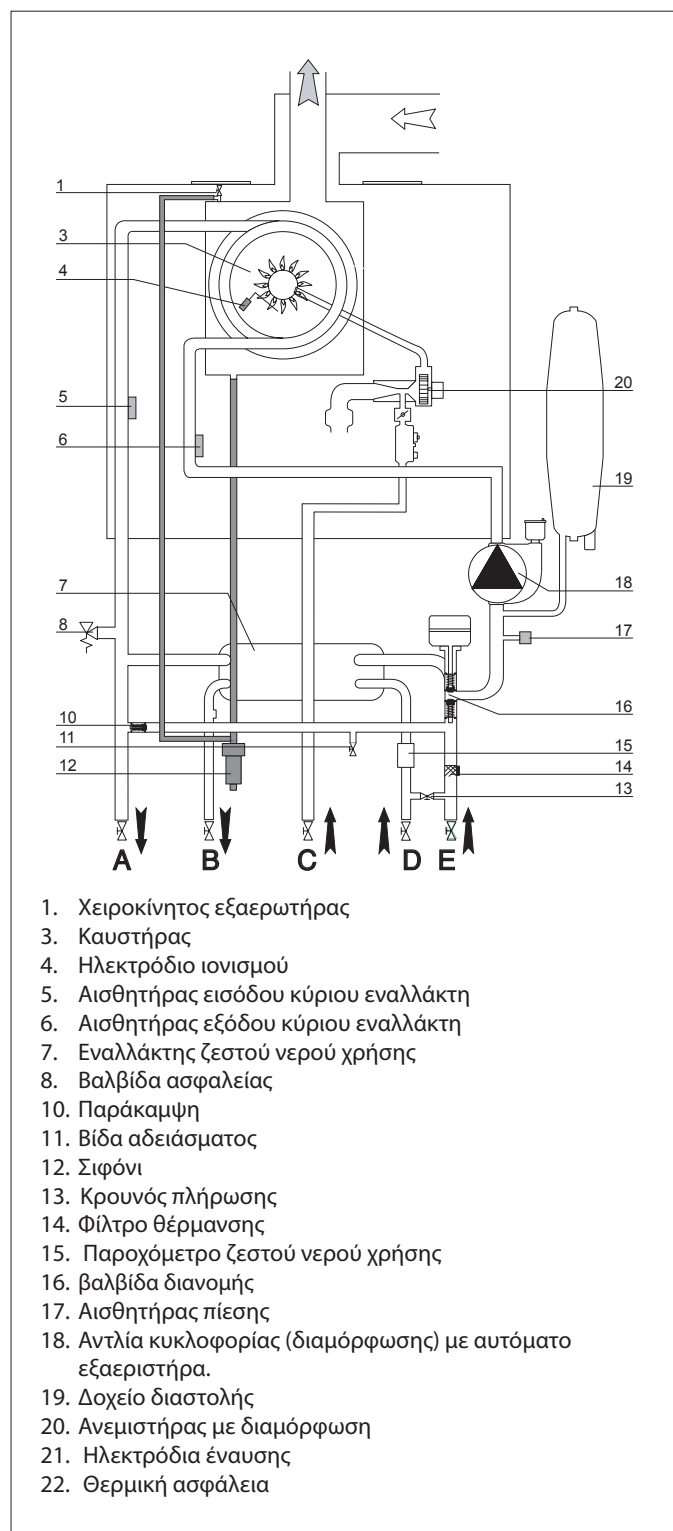
Υδραυλικό σχεδιάγραμμα
